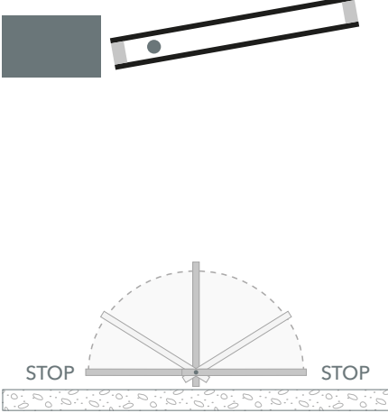
PAIO 2 | Doppio vetro
