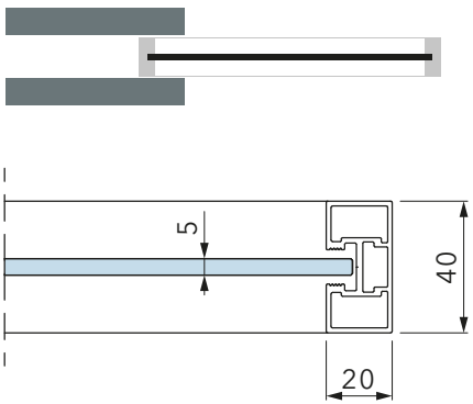
BORA | Singolo vetro
