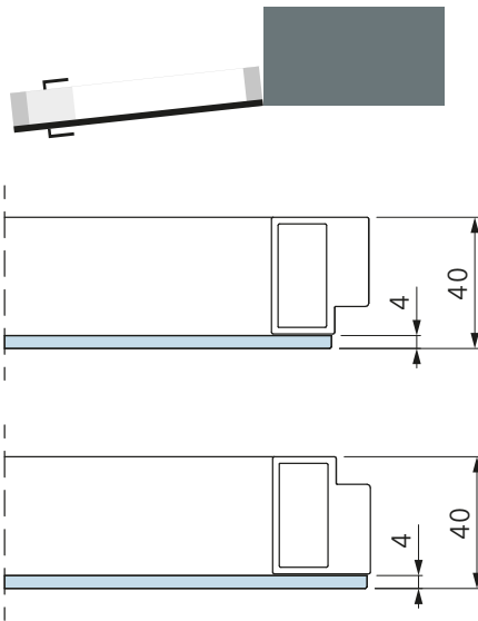
PAIO 1 | Singolo vetro
