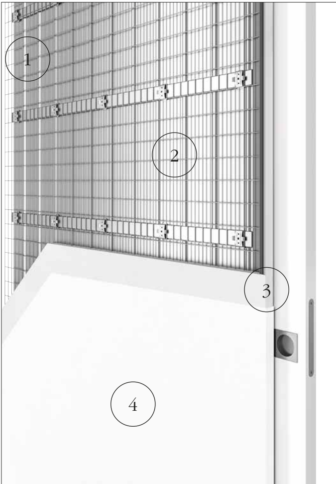
Telaio ECLISSE Syntesis Line Scorrevole - versione intonaco
