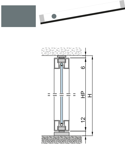
PAIO 1 | Singolo vetro
