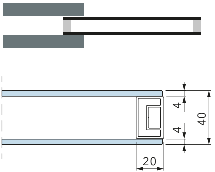
PAIO 2 | Doppio vetro
