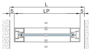
Distanza porta/muro
