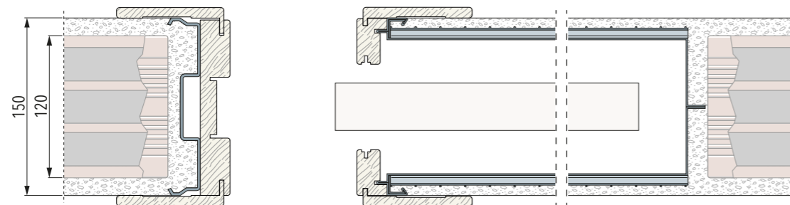
Parete Finita 150 mm - Tramezza 120 mm
