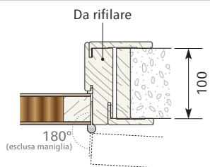
SP 100 mm (stipite da rifilare)
