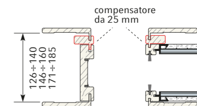
Compensatore da 25 mm
