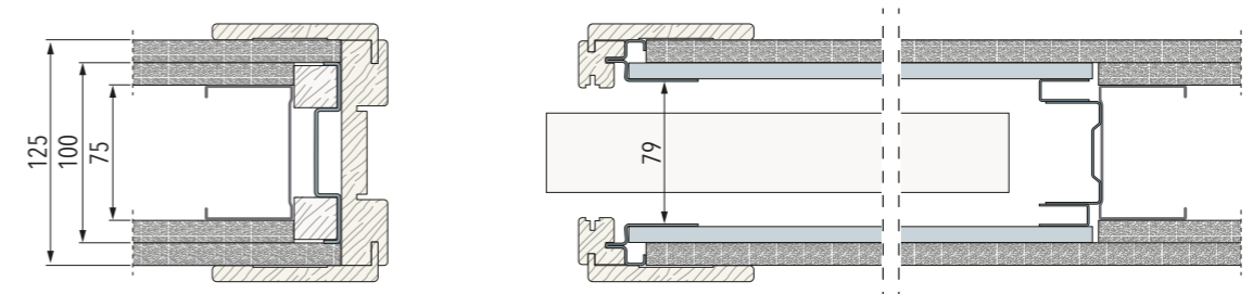
Lastra singola su cassone: Parete Finita 125 mm - Orditura 75 mm | Controtelaio e stipiti da 125 mm
