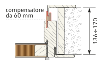
Compensatore da 60 mm
