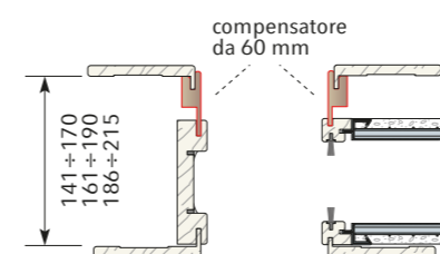
Compensatore da 60 mm
