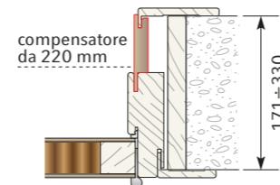
Compensatore da 220 mm
