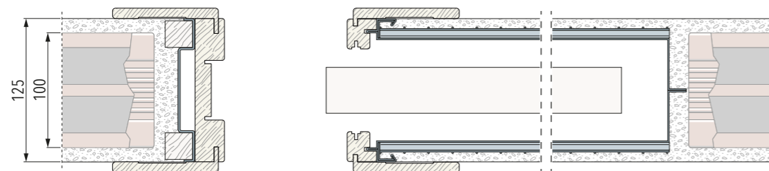
Parete Finita 125 mm - Tramezza 100 mm
