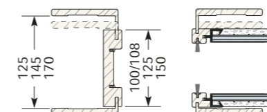
Compensatore da 60 mm
