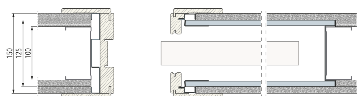
Lastra singola su cassone: Parete Finita 150 mm - Orditura 100 mm | Controtelaio e stipiti da 150 mm
