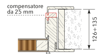
Compensatore da 25 mm
