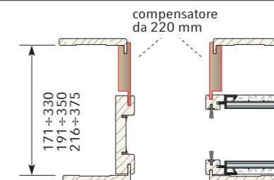
Compensatore da 220 mm
