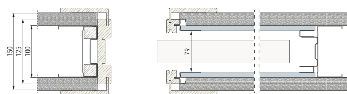
Lastra doppia: Parete Finita 150 mm - Orditura 100 mm | Controtelaio e stipiti da 125 mm
