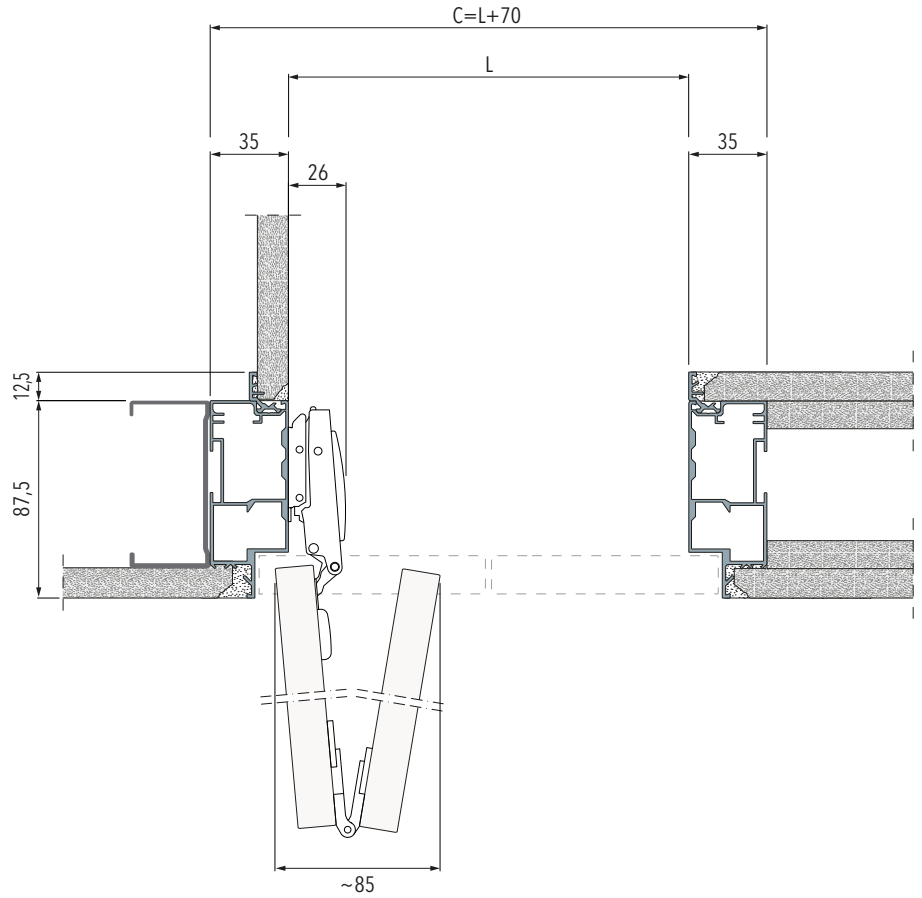
ANTA A LIBRO
