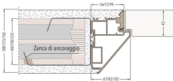
PORTA A SPINGERE
