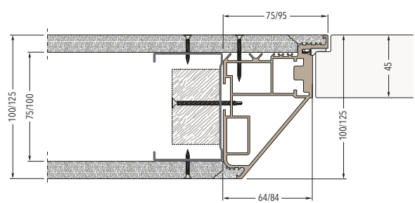
Lastra doppia: Parete finita 125 mm
