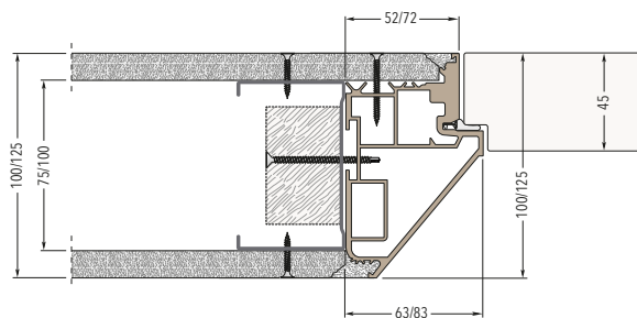
Lastra doppia: Parete finita 125 mm
