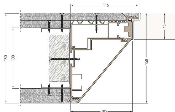
Lastra doppia: Parete finita 150 mm
