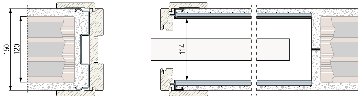
Parete Finita 150 mm - Tramezza 120 mm
